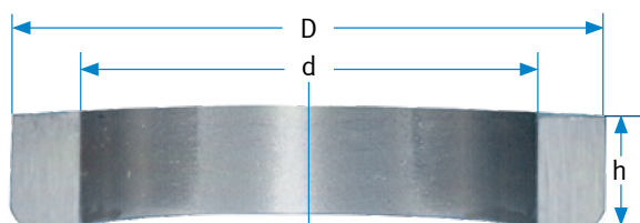
Основные размеры кольца седла клапана
